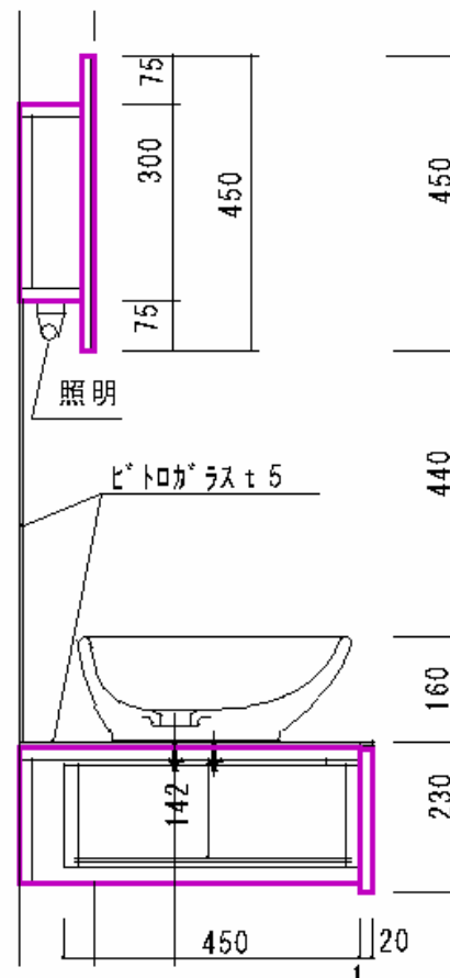
左側断面図
