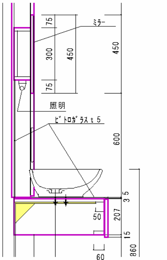
中央断面図
