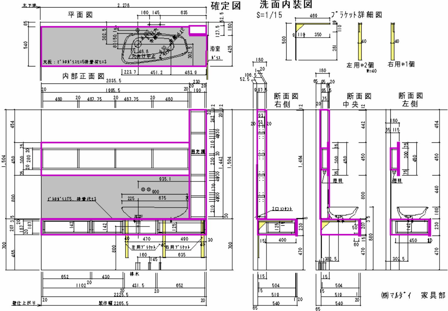
中央断面図
