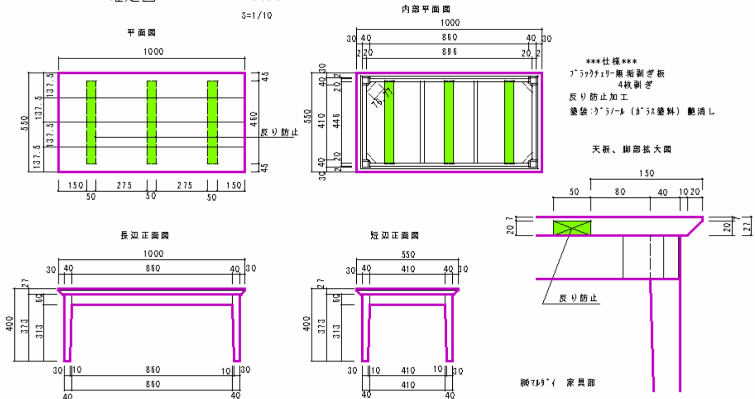
確定図 ブラックチェリー4枚剥ぎ リビングテーブル
