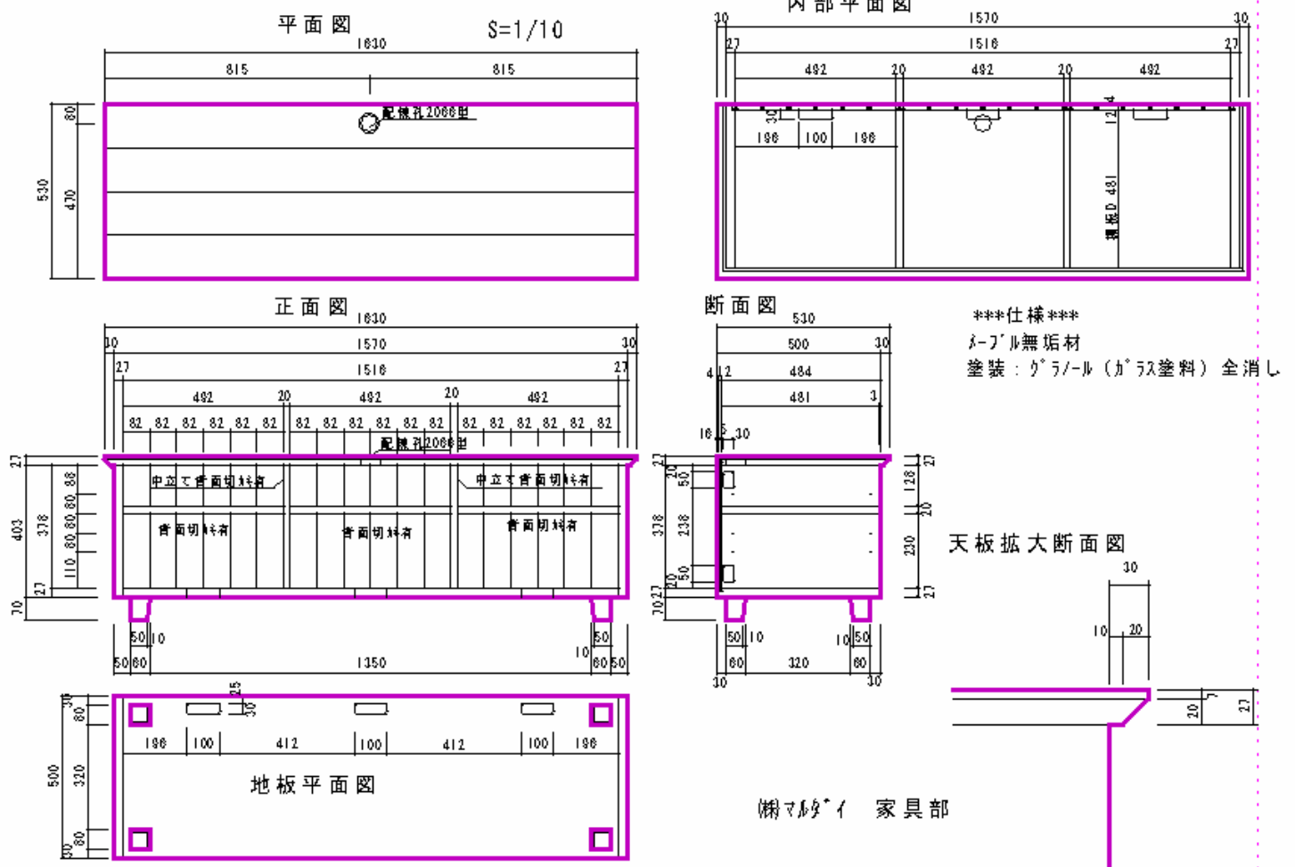
確定図 ハードメープル リビングボード
