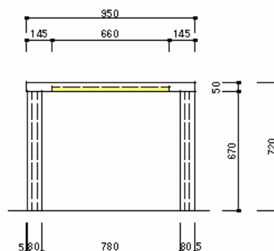
短辺断面図
