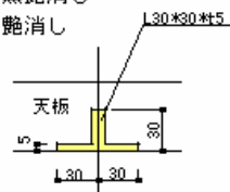
短辺断面図
