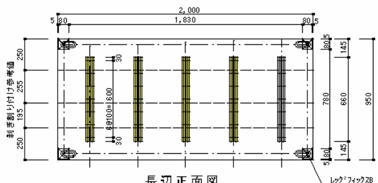
長辺正面図
