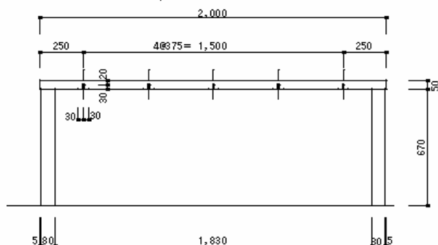
長辺正面図
