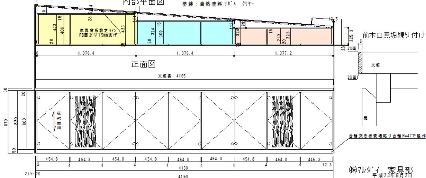
内部平面図
