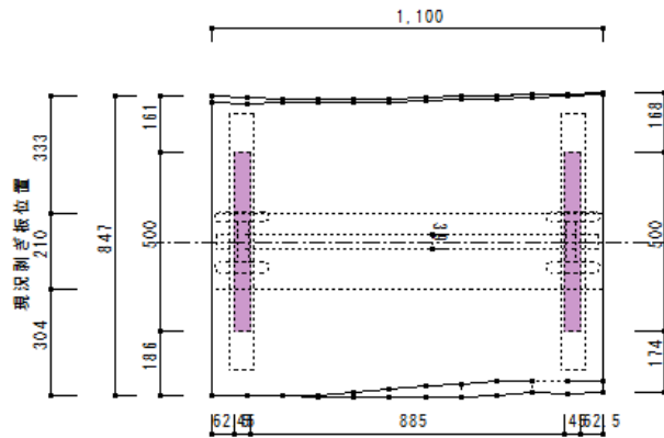
長辺正面図
