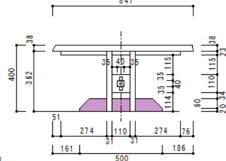
短辺正面図
