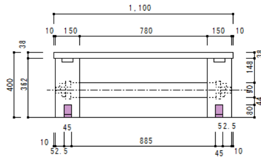
長辺正面図
