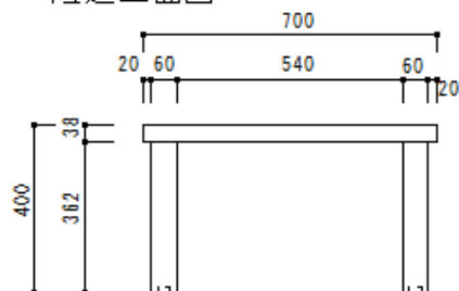
短辺正面図
