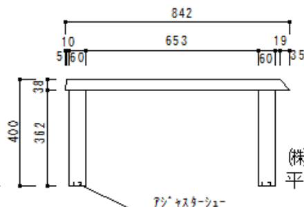
長辺正面図
