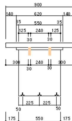
断面図
