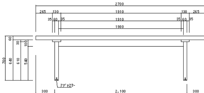
長辺正面図
