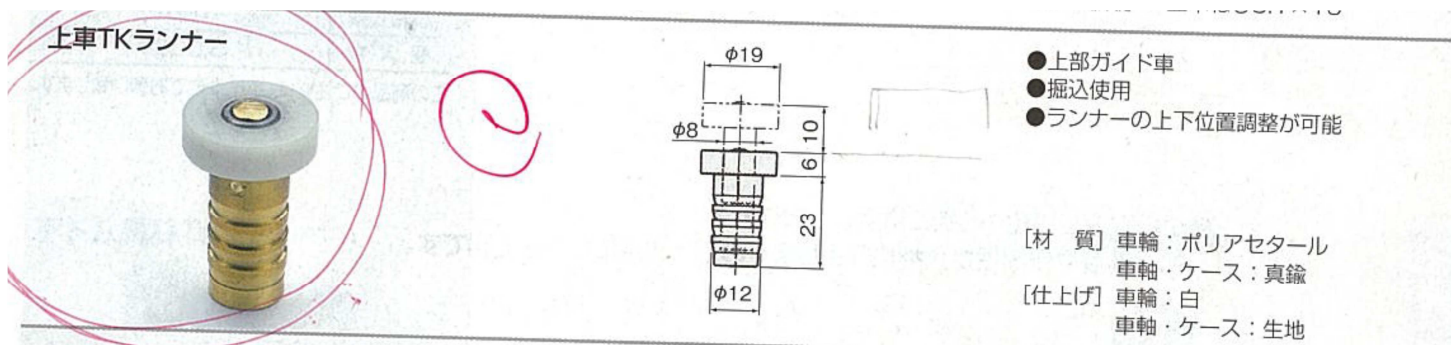
上車 TK ランナー
