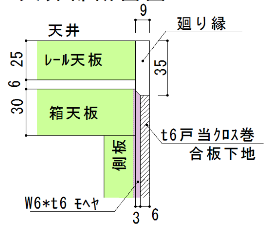
天井部断面図
