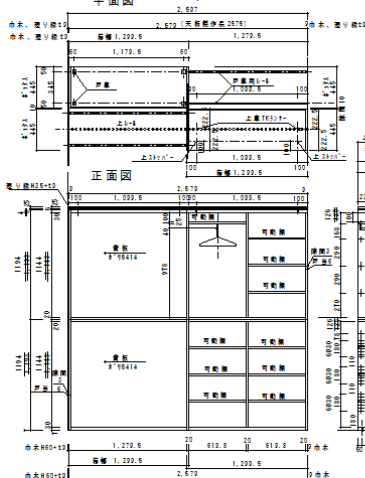
平面図
