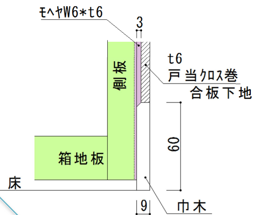
床部断面図
