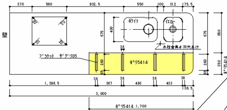
裏平面図
