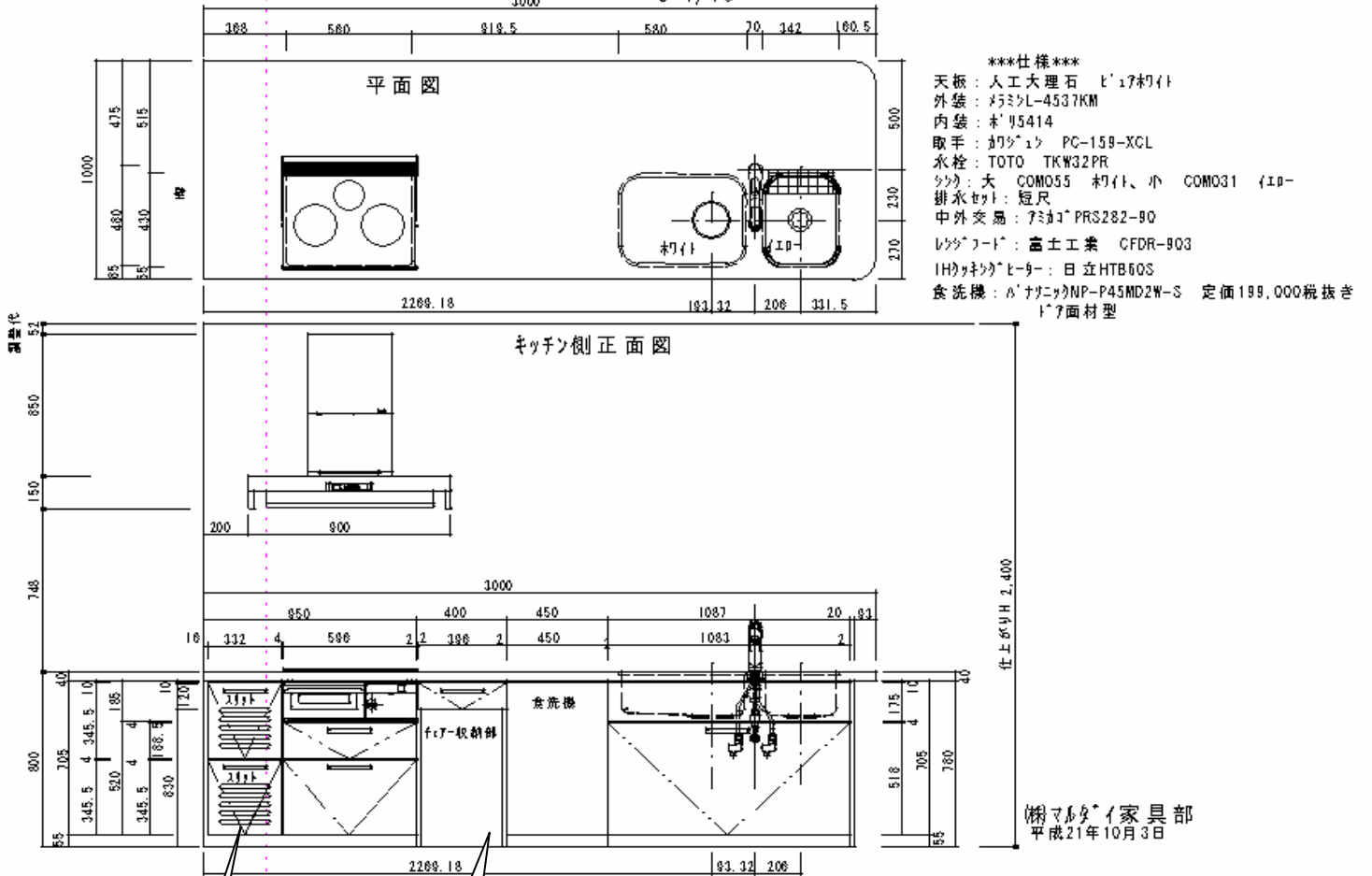
確定図 アイランドキッチン 外装図 S=1/15
