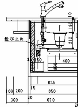
シンク部断面図
