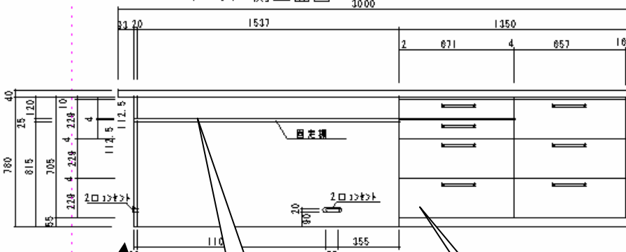
リビング側正面図
