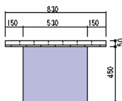
短辺正面図
