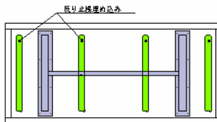
短辺正面図
