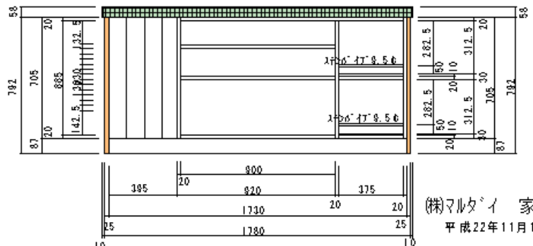
背面図
