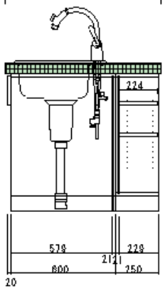
背面図
