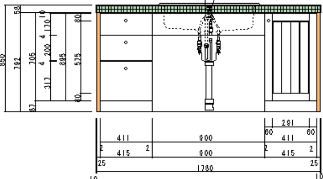
正面図
