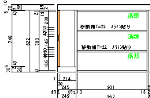
キッチン側正面図
