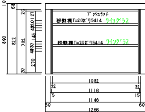
タイル側内部正面図
