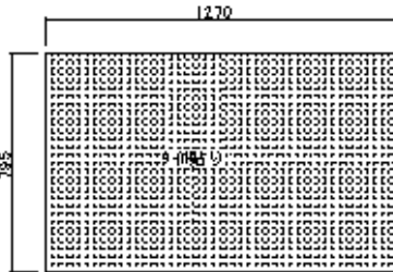
タイル側正面図
