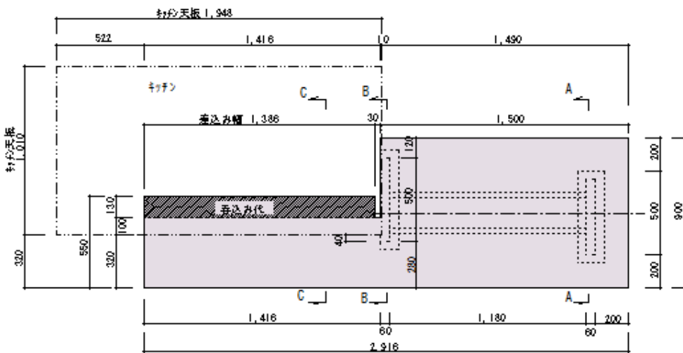
1月18日 確定図 キッチン部+ダイニングカウンター 平面図 S=1/15
