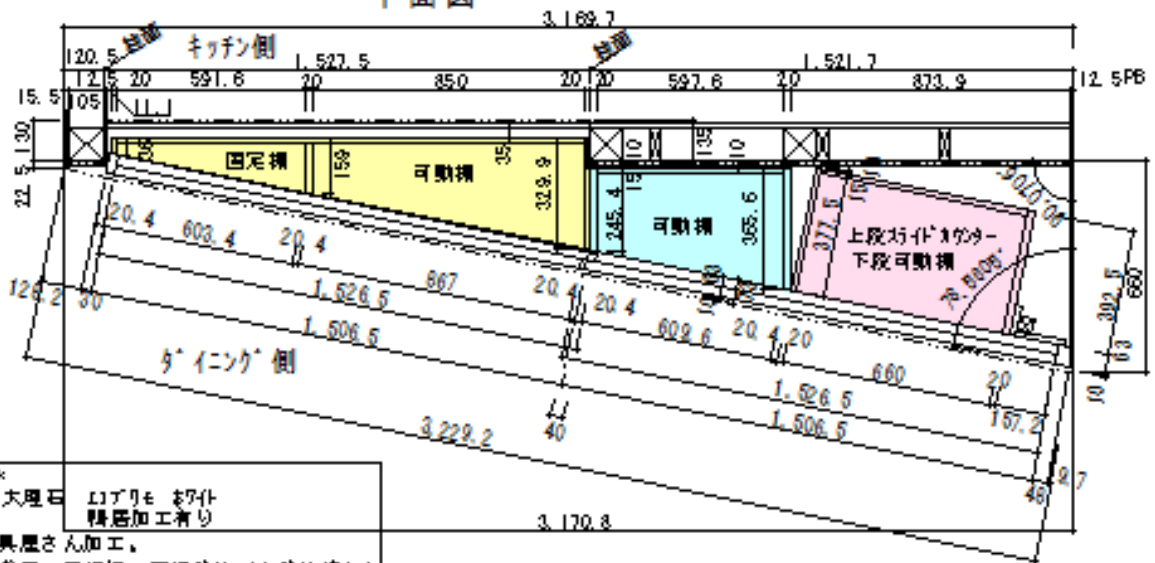
平面図
