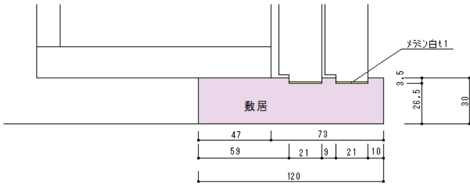
敷居平面図
