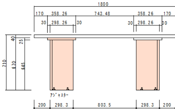
長辺正面図
