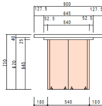
短辺正面図
