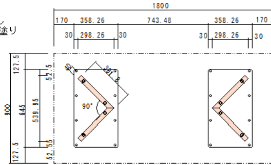
脚部平面図
