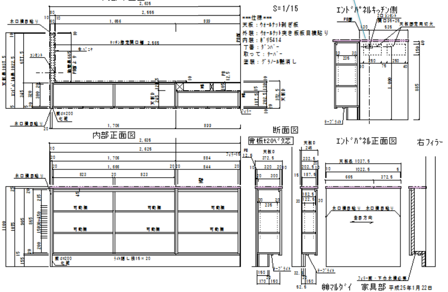
内部平面図 1/22 確定図 キッチンカウンター収納内装図
