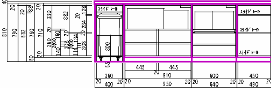
内部正面図
