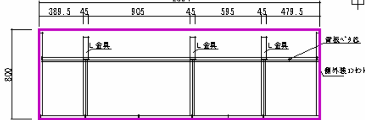
正面図
