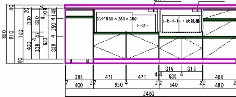
内部正面図
