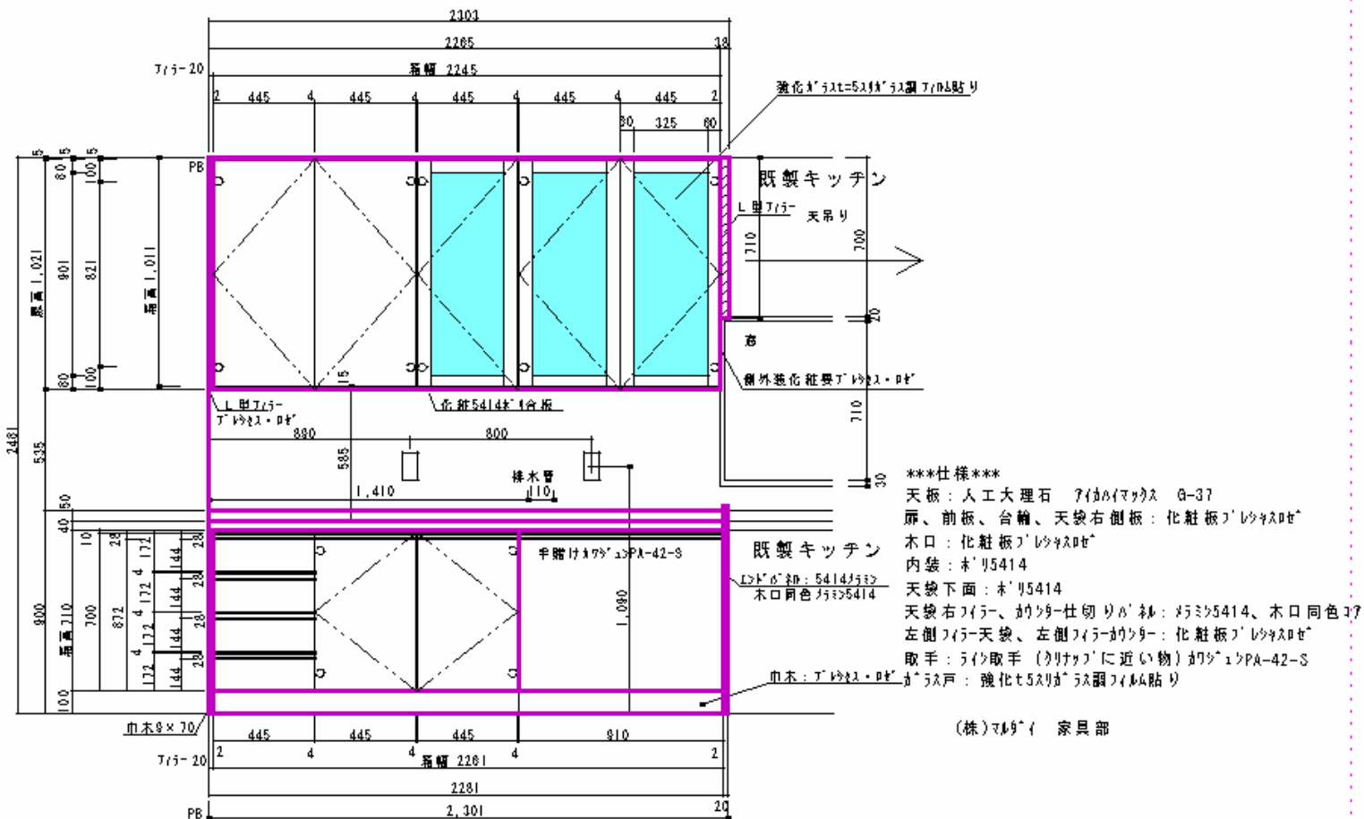
キッチン横収納外装図
