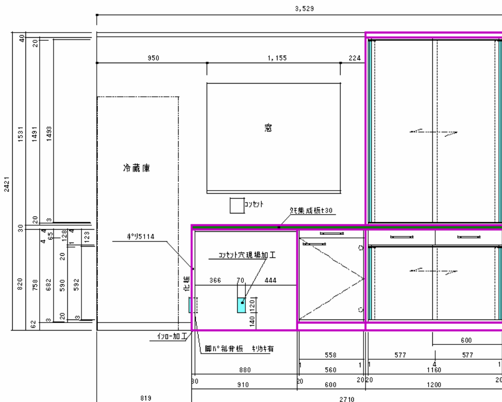
確定図 キッチン背面収納 正面図
