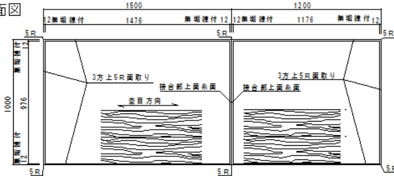
天板平面図
