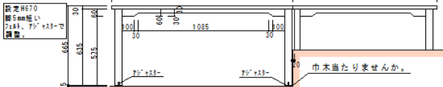
長辺正面図
