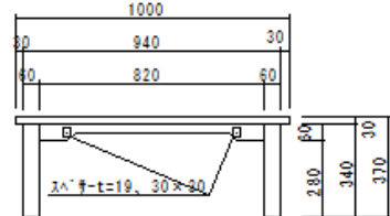
接合面短辺正面図
